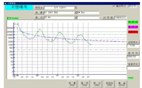
수명예측 각 감시CABLE의 향후 절연저항 변화예측 및 잔존수명예측
