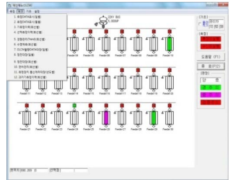
MENU화면 계통도에 감시CABLE의 절연상태를 색상으로 표시되므로 양호, 불량 판별 용이 및 MENU표시
